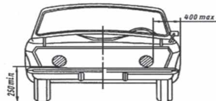
Правила установки противотуманных фар
